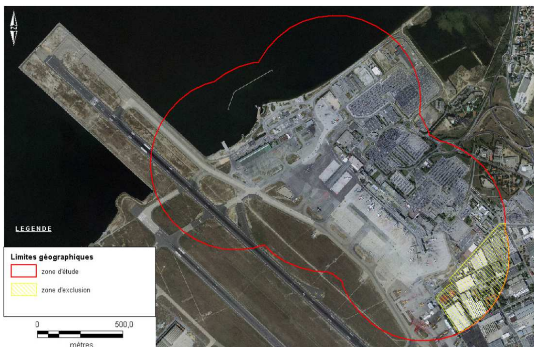
Ortho-photo de l'aéroport de Marseille Provence (AMP) présentant la zone d'étude du RSI. La zone hachurée en jaune représente la zone située en dehors des limites administratives de l'aéroport.
